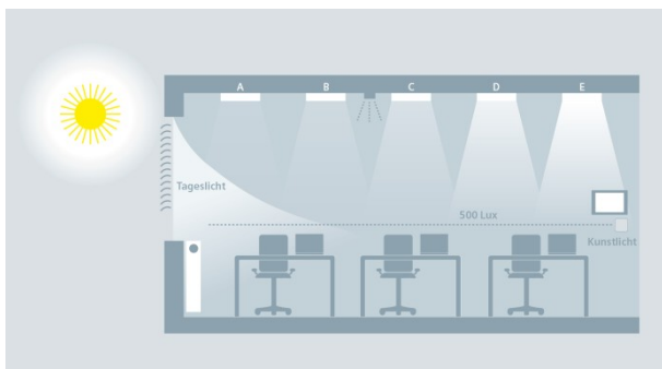
Abb. 4 Prinzip einer Konstantlichtregelung bei fünf Leuchtengruppen
