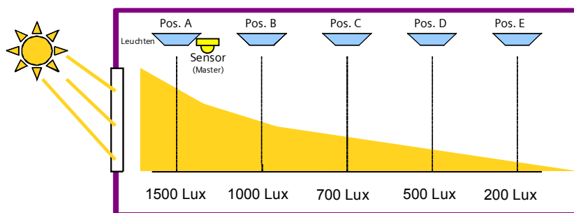
Abb. 9 Helligkeitsverteilung des Tageslichts nach Raumtiefe
