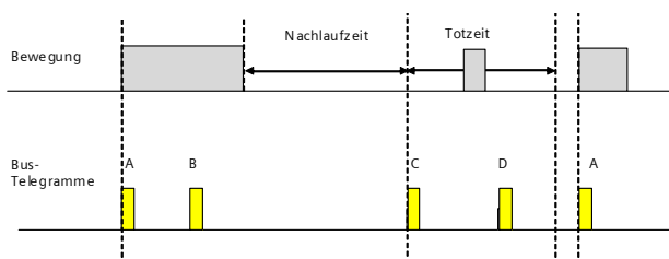
Abb. 2 Ablaufdiagramm
