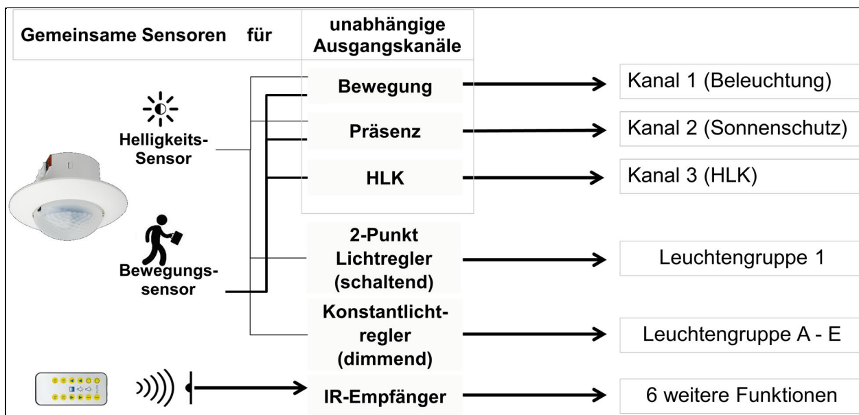
Abb. 1 Drei unabhängig konfigurierbare Ausgangskanäle für verschiedene Anwendungen
