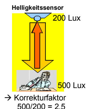
Abb. 8 indirekte Messung
