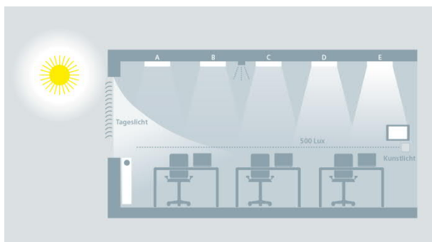
Abb. 4 Prinzip einer Konstantlichtregelung bei fünf Leuchtengruppen
