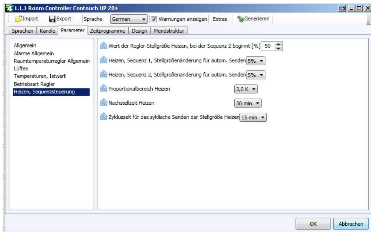
Abb. 62. Parameteransicht: Heizen, Sequenzsteuerung
