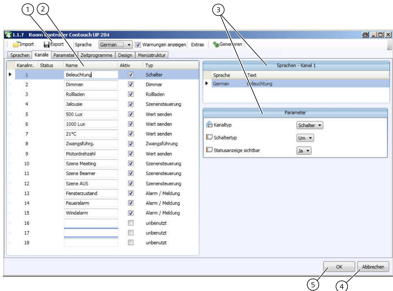
Abb. 6. Arbeitsbereich des Contouch Manager (Bsp. Konfigurationsfenster Kanäle)
