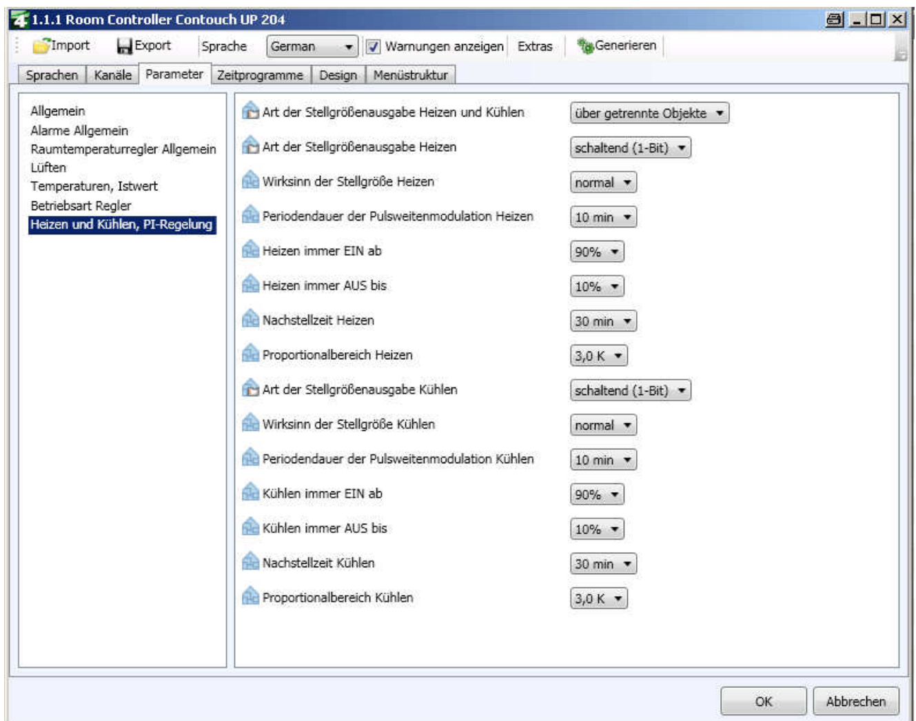
Abb. 66. Parameteransicht: Heizen und Kühlen, PI-Regelung
