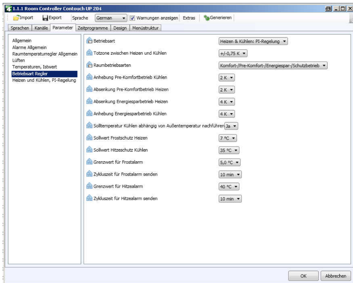
Abb. 59. Parameteransicht: Betriebsart Regler
