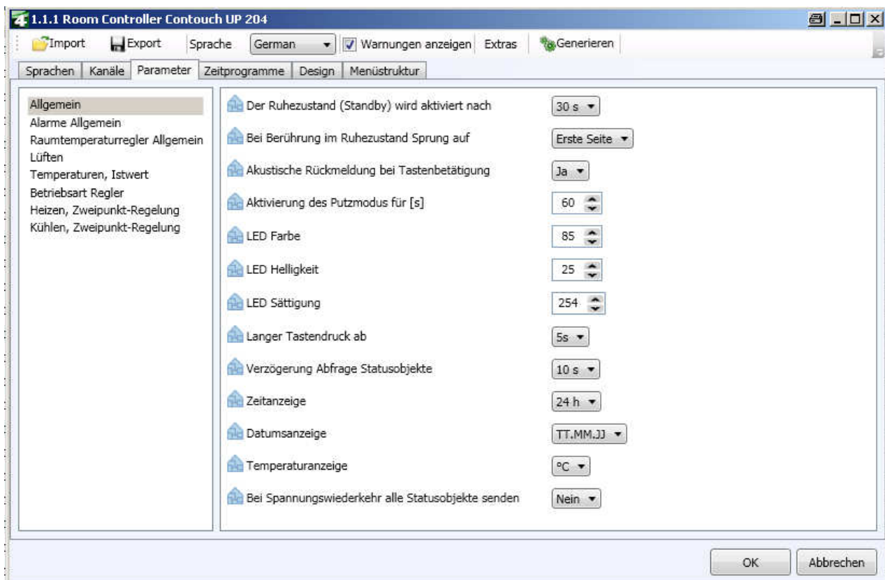
Abb. 54. Parameteransicht: Allgemein
