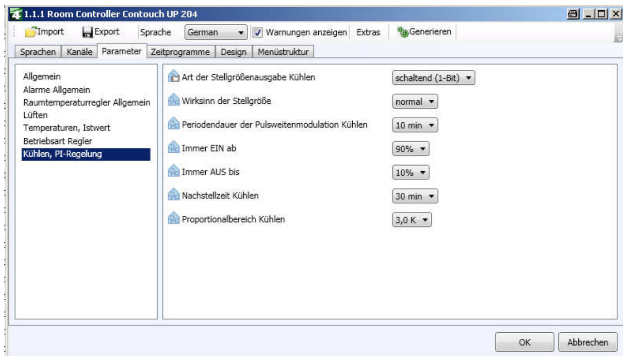
Abb. 64. Parameteransicht: Kühlen, PI-Regelung
