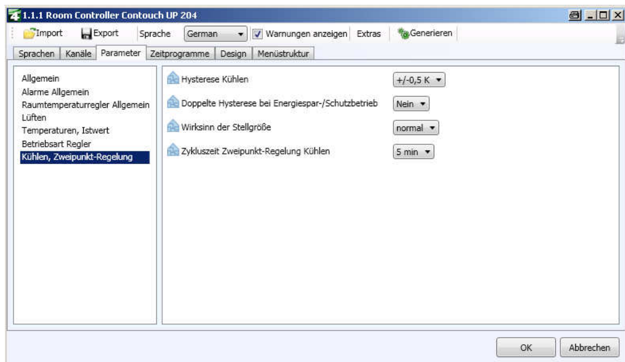
Abb. 63. Parameteransicht: Kühlen, Zweipunkt-Regelung
