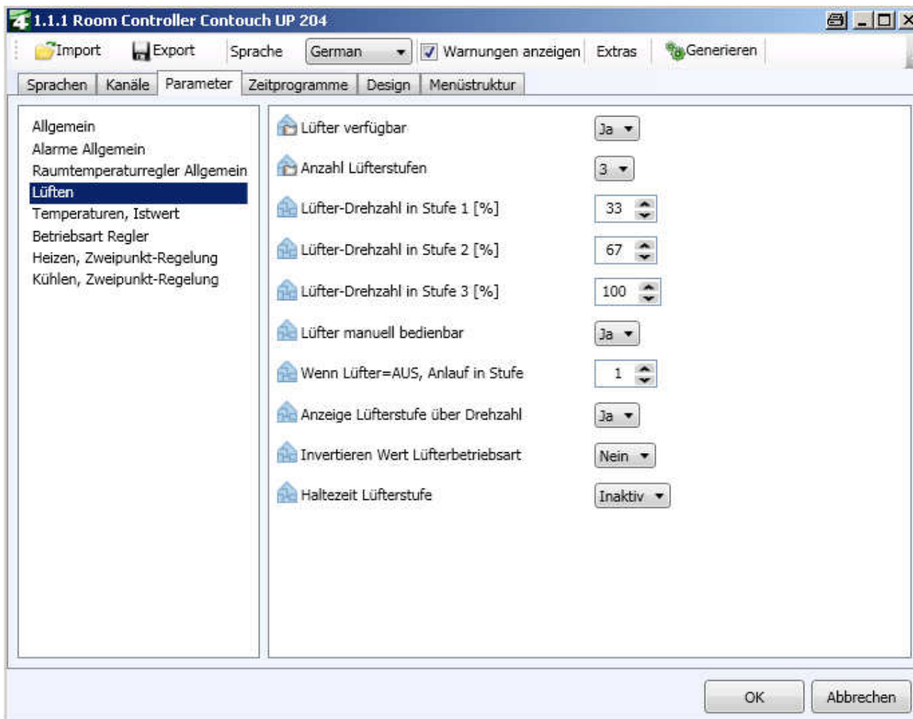
Abb. 57. Parameteransicht: Lüften
