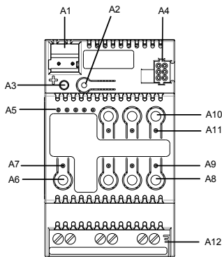
Bild 2: Anzeigeelemente und Bedienelemente
