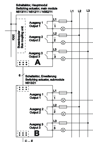
Bild 1: Schaltaktor-Hauptmodul und -Erweiterung
