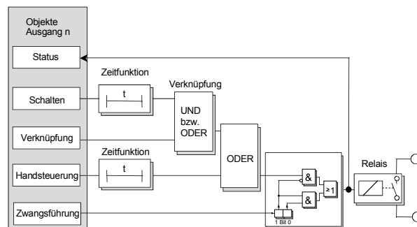
Bild 3: Blockschaltbild eines Ausgangs im Normalbetrieb
