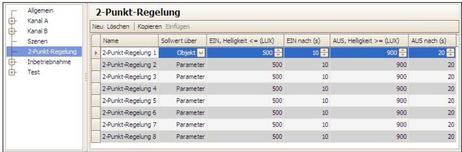
Abb. 28 Parameterfenster 2-Punkt-Regelung
