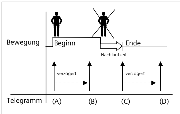
Abb. 19 Telegrammfolge Präsenzmelder
