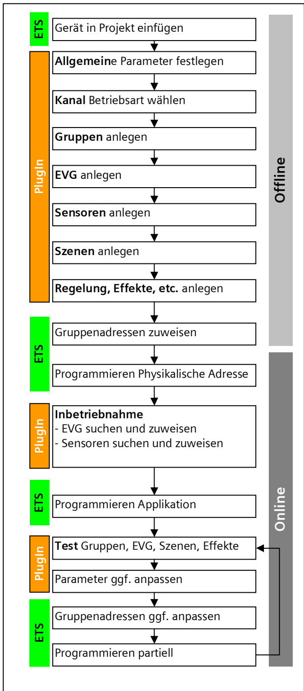
Abb. 1 Konfigurationsschritte
