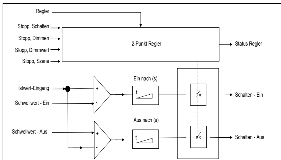
Abb. 27 Funktionsblock 2-Punkt-Regelung
