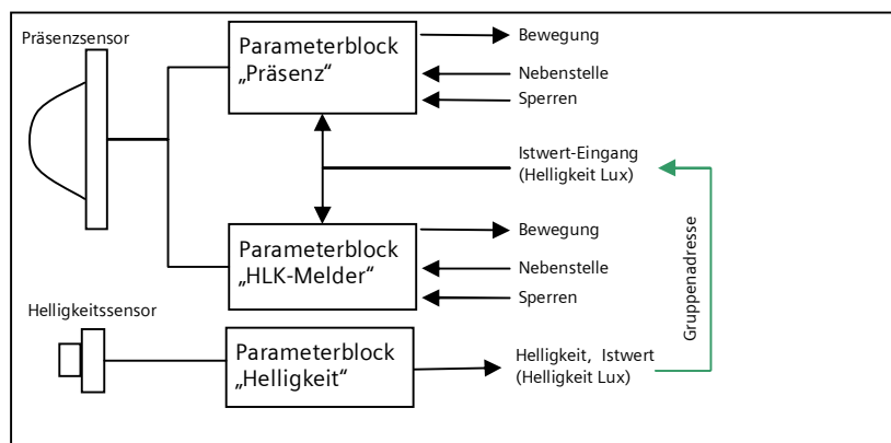
Abb. 18 Funktionsblöcke
