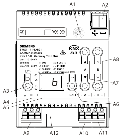
Abb. 45 Bedien- und Anzeigeelemente Gateway
