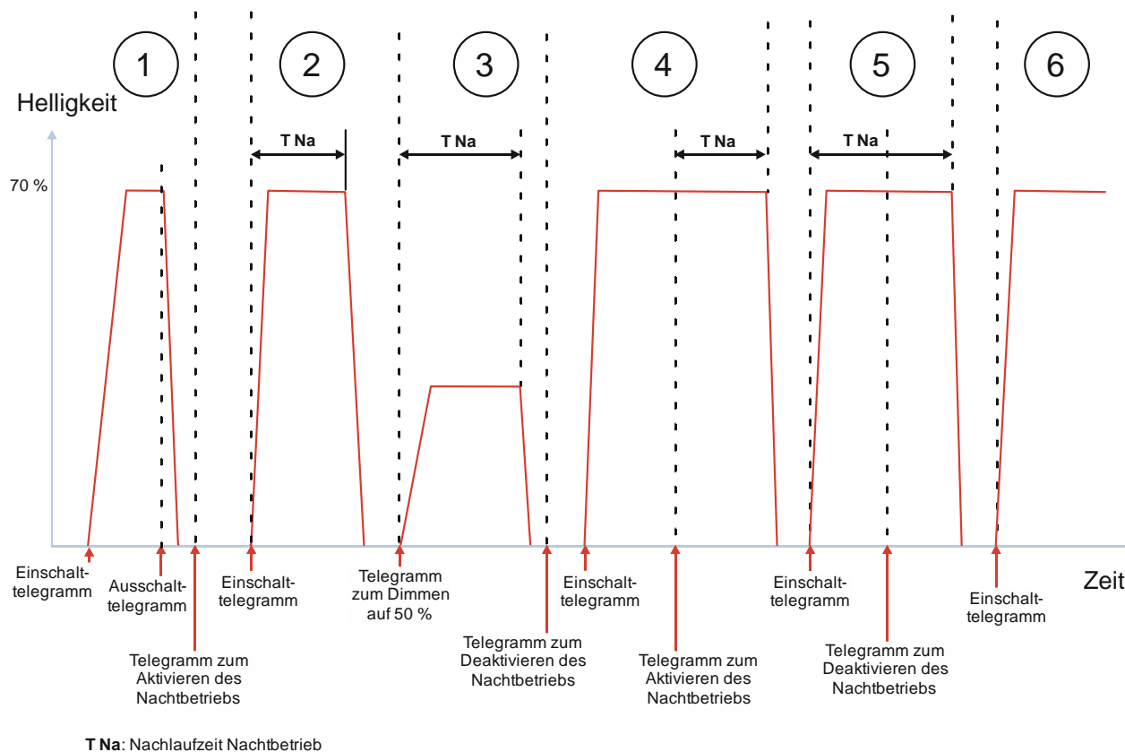
Abb. 45 Verhalten bei Aktivierung und Deaktivierung des Nachtbetriebs im Normalbetrieb
