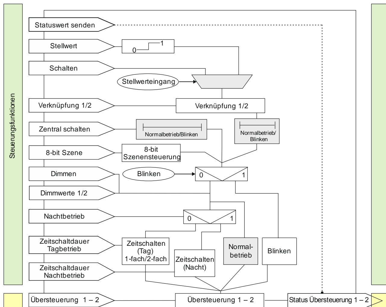
Abb. 3 Normalbetrieb
