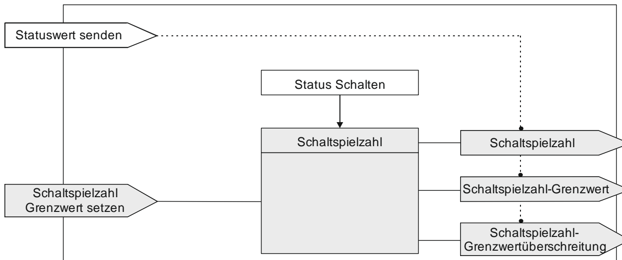
Abb. 20 Schaltspielzählung (Details)
