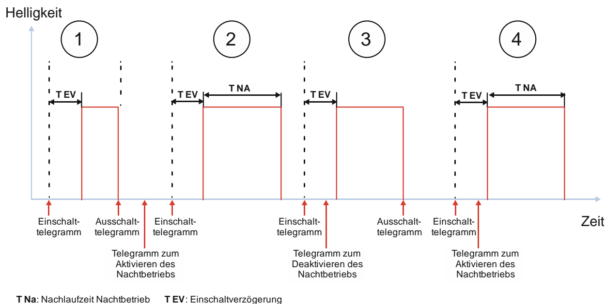
Abb. 49 Verhalten bei parametrierter Einschaltverzögerung im Normalbetrieb und Nachtbetrieb
