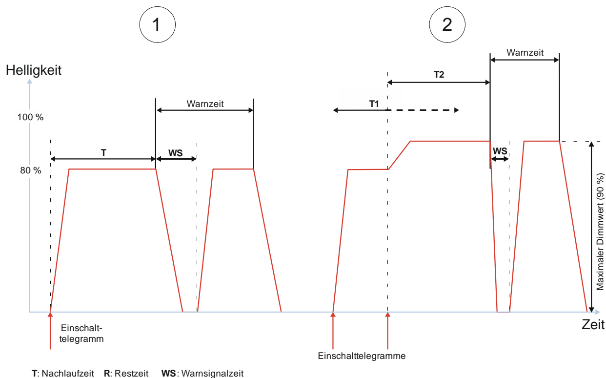
Abb. 41 Verhalten bei Zeitschalterbetrieb (1-fach) mit Einstellung „Warnen vor Ausschalten“ = „kurzes Aus-/Einschalten“ und „Nachtriggern möglich“ = „1“
