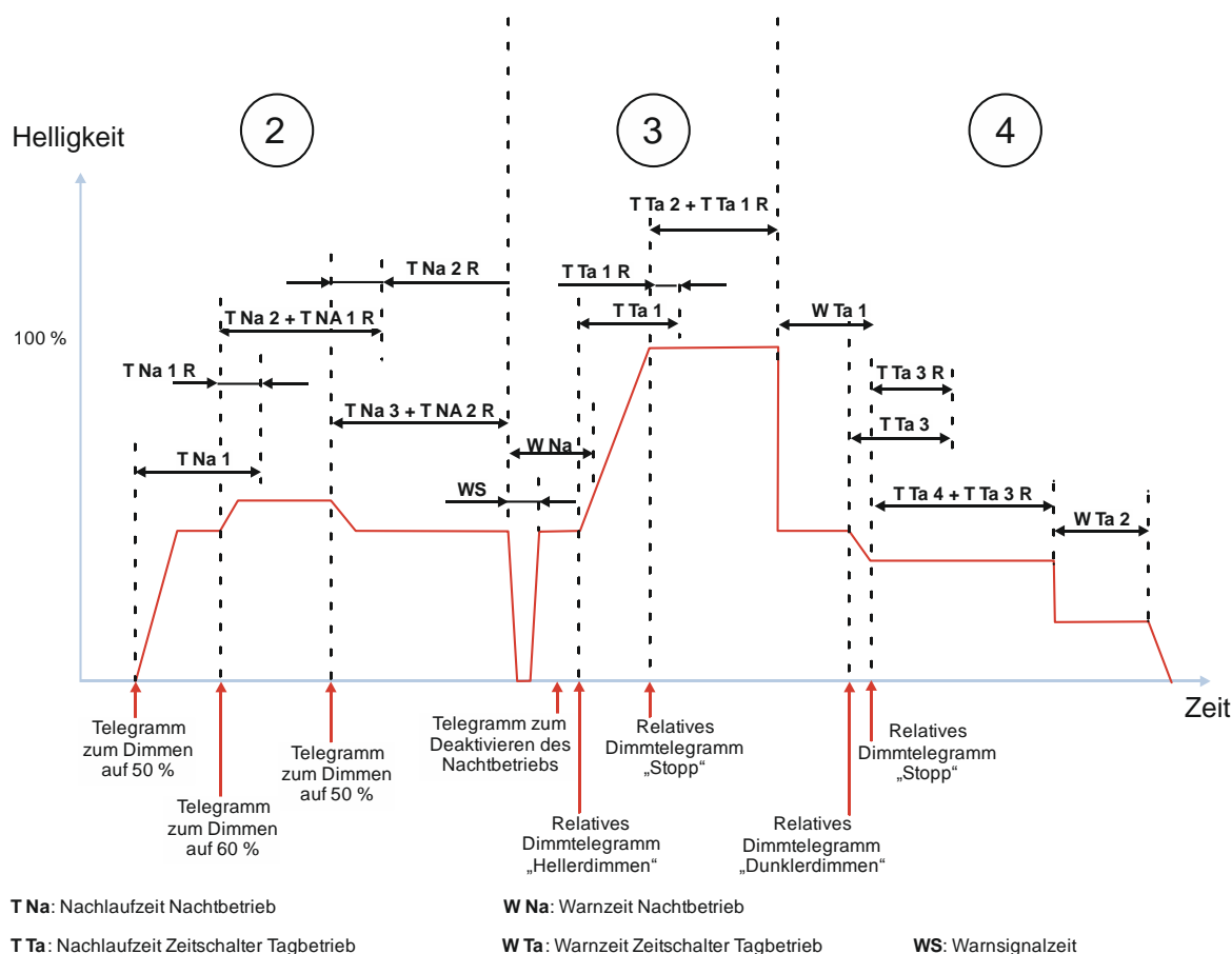
Abb. 48 Verhalten bei Aktivierung und Deaktivierung des Nachtbetriebs im Zeitschalterbetrieb (1-fach)
