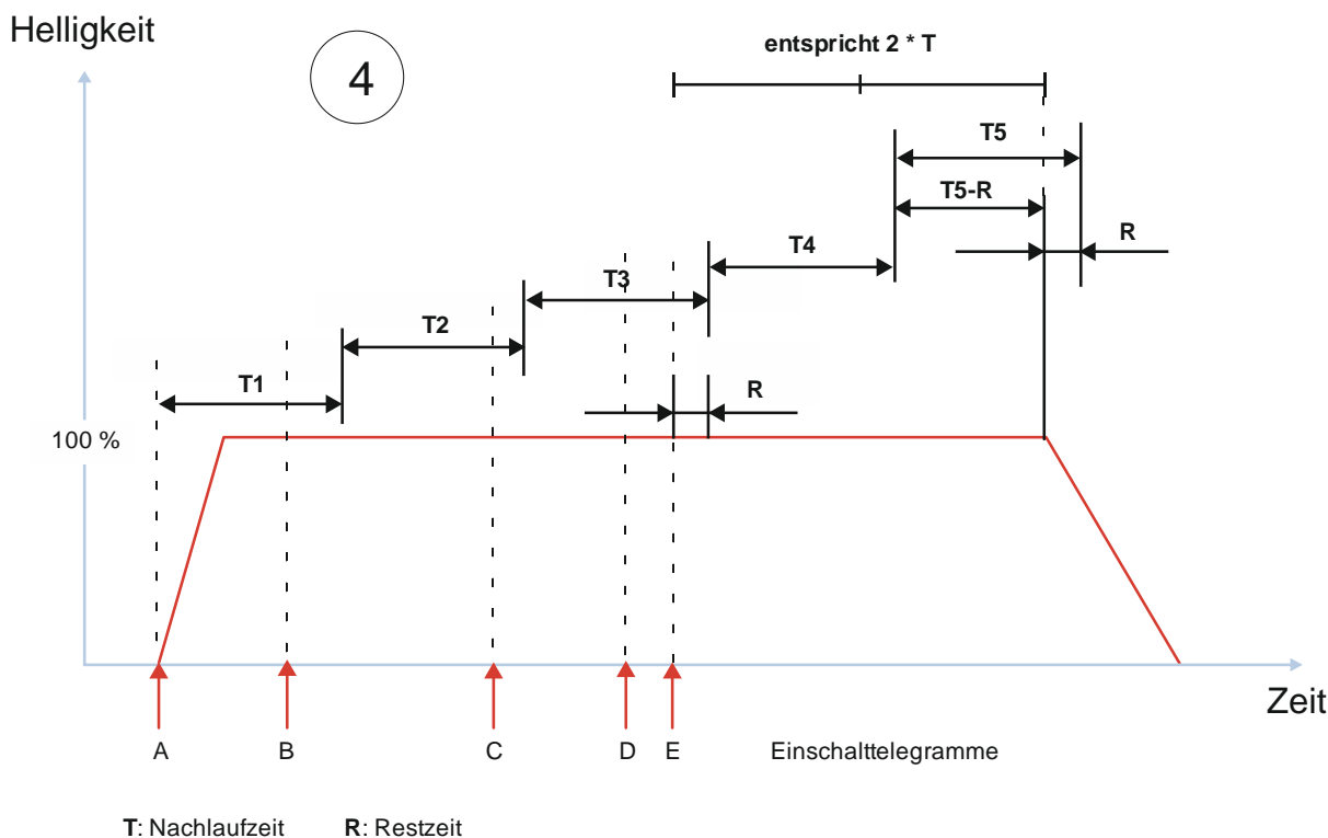
Abb. 40 Verhalten bei Zeitschalterbetrieb (1-fach) mit Einstellung „Nachtriggern möglich“ = „2“
