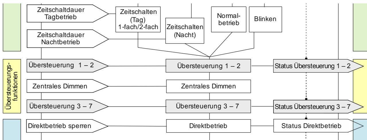
Abb. 11 Übersteuerungen
