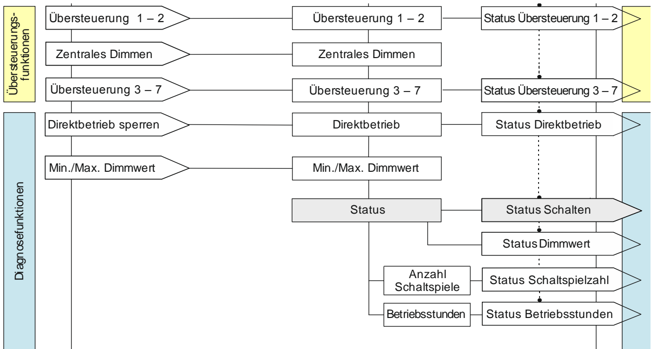
Abb. 18 Status
