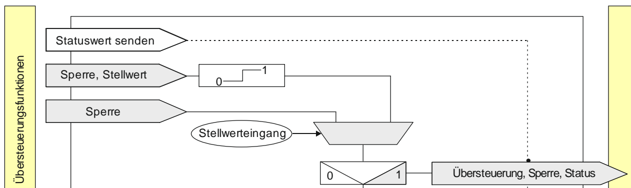
Abb. 14 Übersteuerung Sperrung Kommunikationsobjekte zur Übersteuerung „Sperrung“
