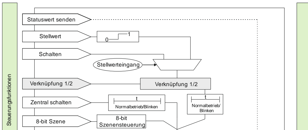
Abb. 6 Logische Verknüpfungen
