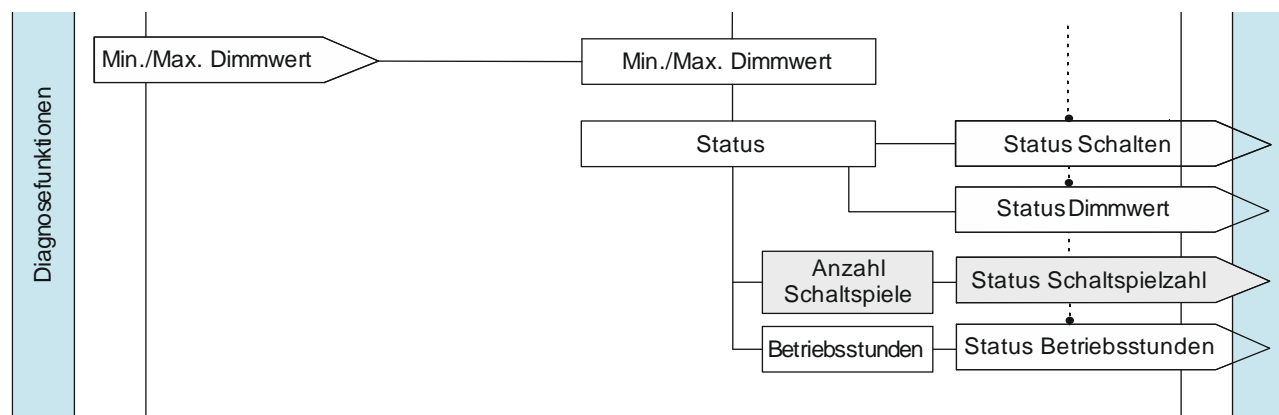
Abb. 19 Schaltspielzählung (Übersicht)
