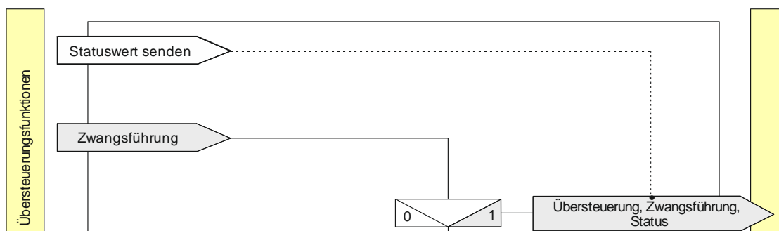
Abb. 17 Zwangsführung
