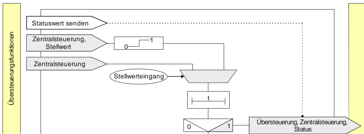
Abb. 15 Zentralübersteuerung
