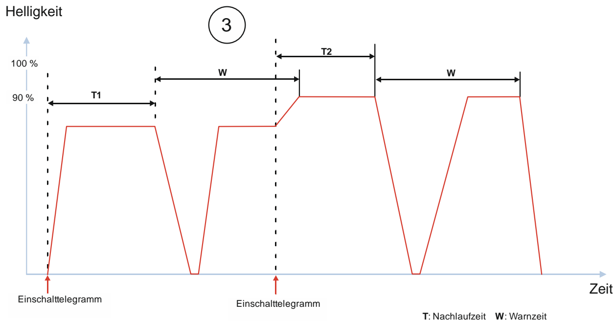
Abb. 42 Verhalten bei Zeitschalterbetrieb (1-fach) mit Einstellung „Warnen vor Ausschalten“ = „kurzes Aus-/Einschalten“ und „Nachtriggern möglich“ = „1“
