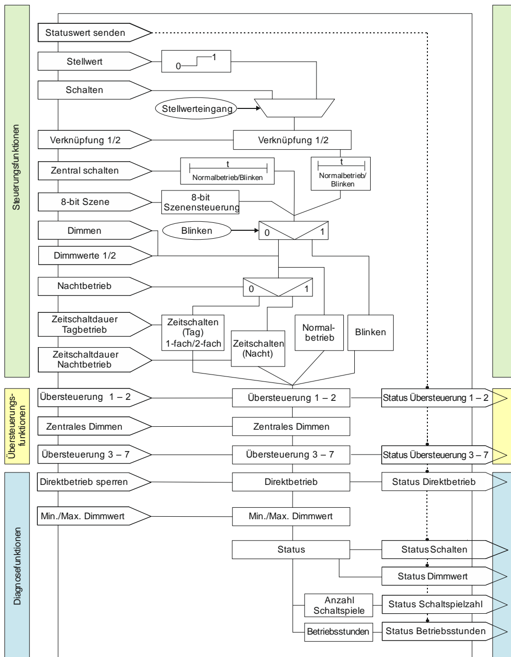
Abb. 1 Schematischer Aufbau eines Dimmerkanals
