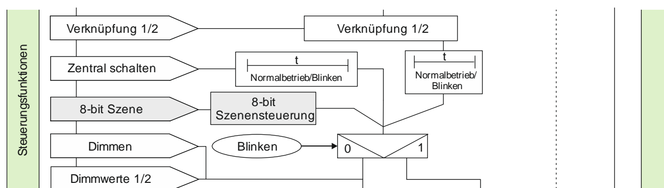
Abb. 9 8-bit Szenensteuerung
