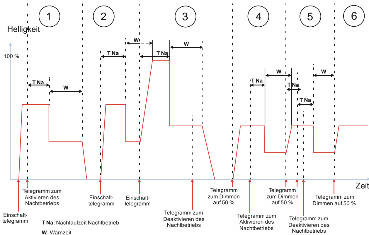
Abb. 46 Verhalten bei Aktivierung und Deaktivierung des Nachtbetriebs im Normalbetrieb mit einer Warnung vor dem Ausschalten
