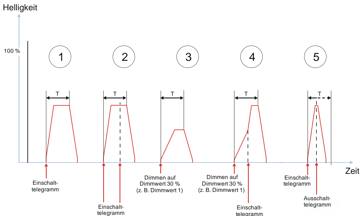
Abb. 37 Verhalten bei Zeitschalterbetrieb (1-fach) mit Einstellung „Nachtriggern = 0“
