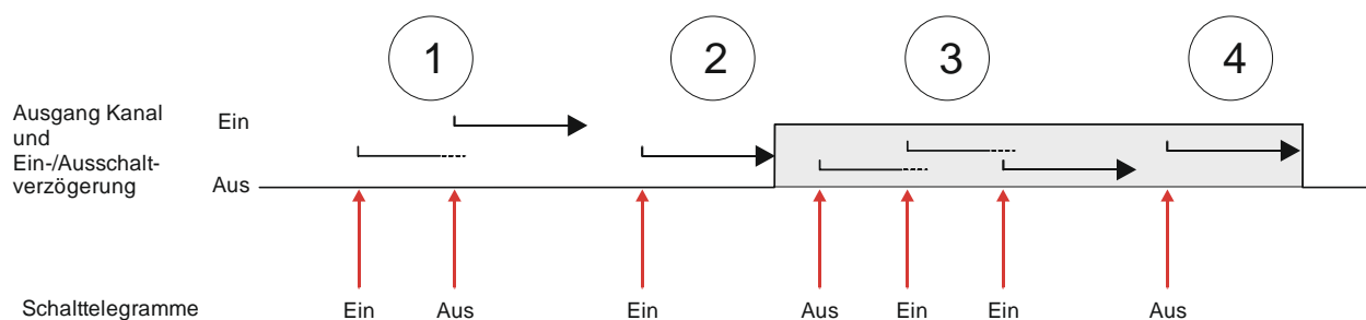
Abb. 36 Schaltverhalten bei parametrierter Ein- und Ausschaltverzögerung
