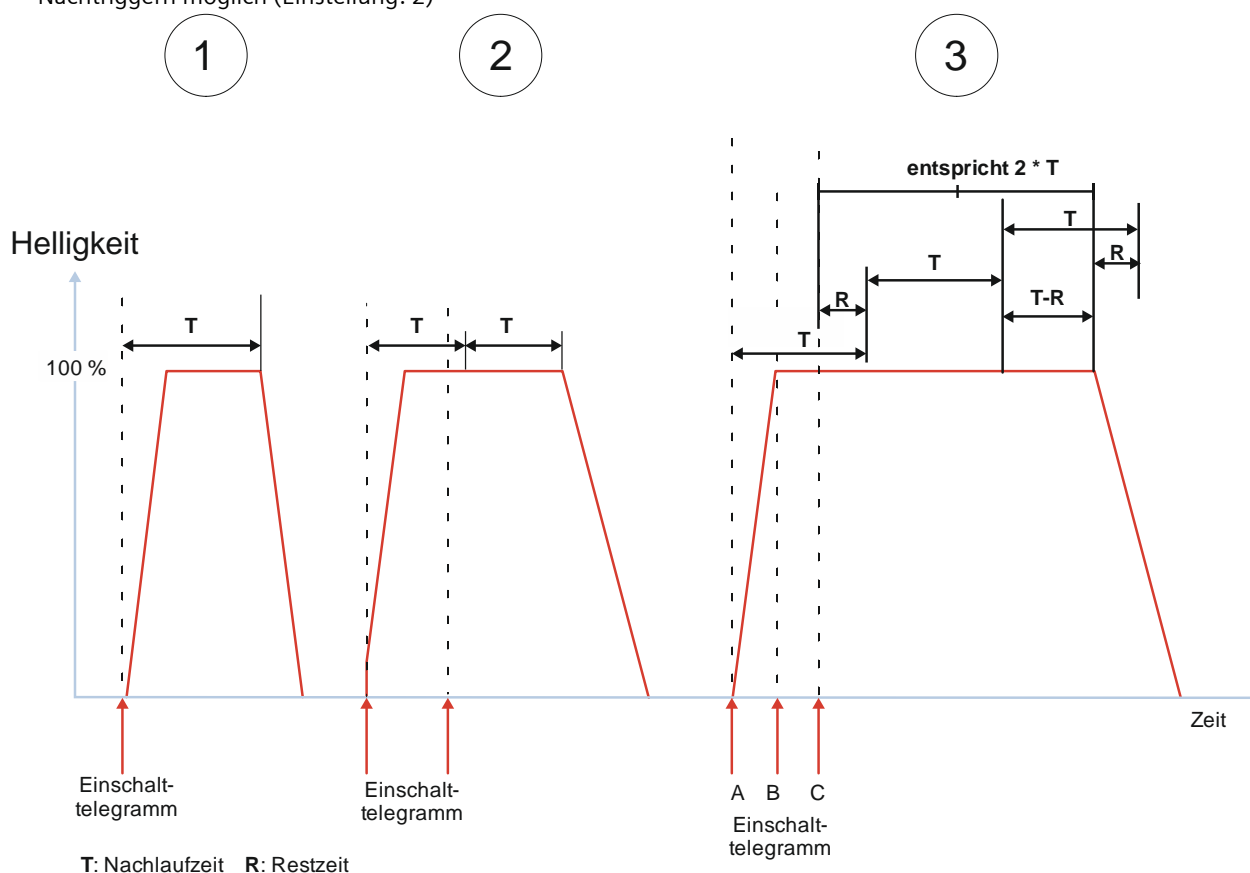
Abb. 39 Verhalten bei Zeitschalterbetrieb (1-fach) mit Einstellung „Nachtriggern möglich“ = „2“
