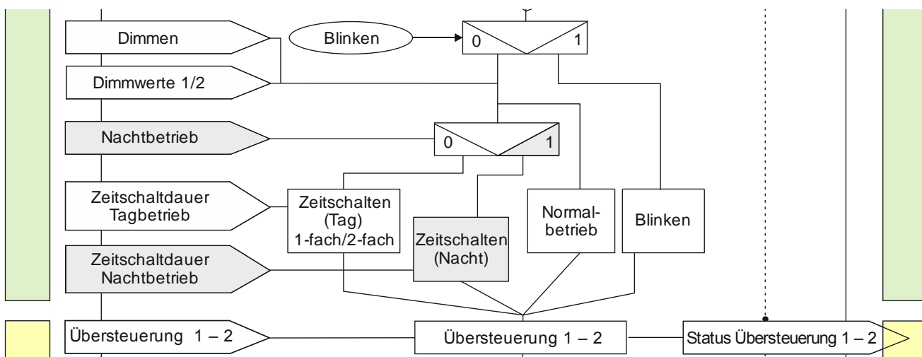
Abb. 10 Nachtbetrieb
