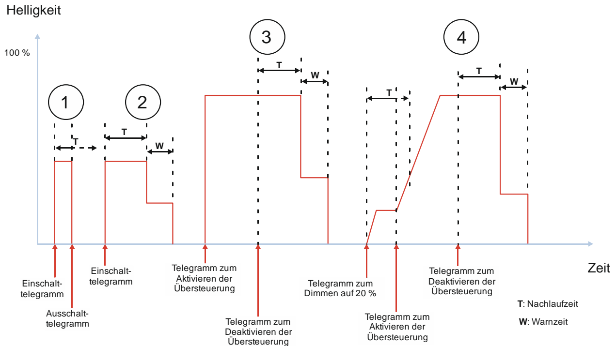
Abb. 52 Verhalten des Schalt-/Dimmaktors im Zeitschalterbetrieb bei parametrierter Übersteuerung (Zwangsführung) und Vorgabe zum Neustart des Zeitschalters bei Deaktivierung der Übersteuerung
