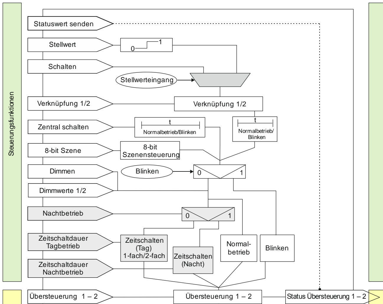
Abb. 4 Zeitschalterbetrieb und Zeitschalterbetrieb 2-fach
