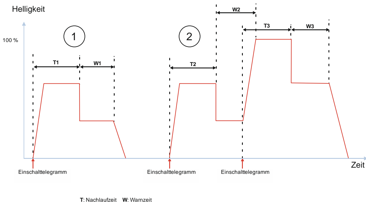
Abb. 43 Verhalten bei Zeitschalterbetrieb (1-fach) mit Einstellung „Warnen vor Ausschalten“ = „durch Dimmen auf den halben Dimmwert“ und „Nachtriggern möglich“ = „1“
