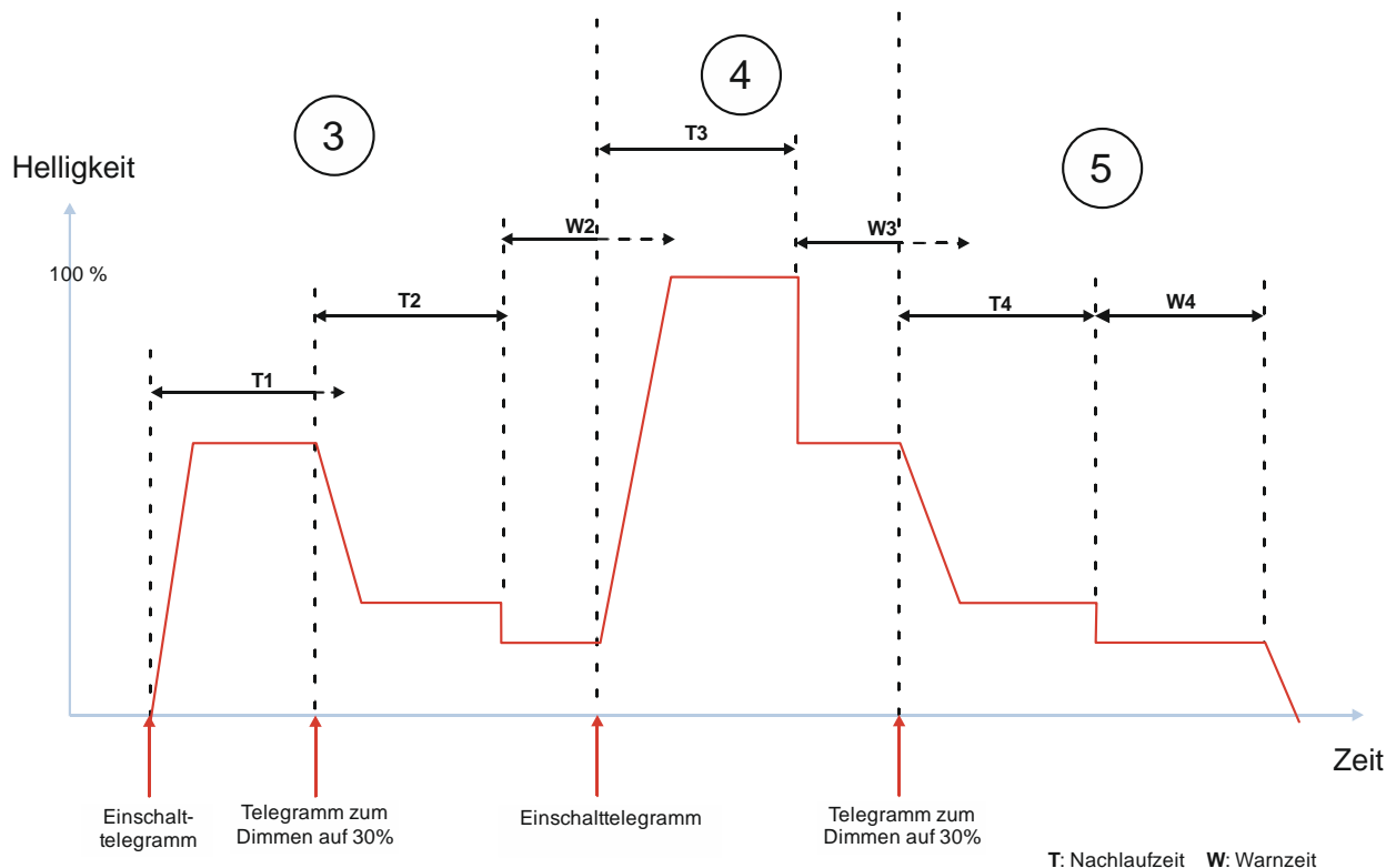
Abb. 44 Verhalten bei Zeitschalterbetrieb (1-fach) mit Einstellung „Warnen vor Ausschalten“ = „durch Dimmen auf den halben Dimmwert“ und „Nachtriggern möglich“ = „1“
