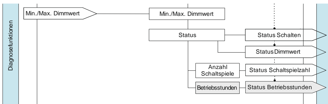
Abb. 21 Betriebsstundenzählung (Übersicht)
