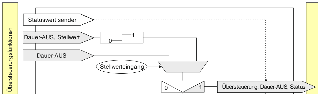
Abb. 13 Übersteuerung „Dauer-AUS“
