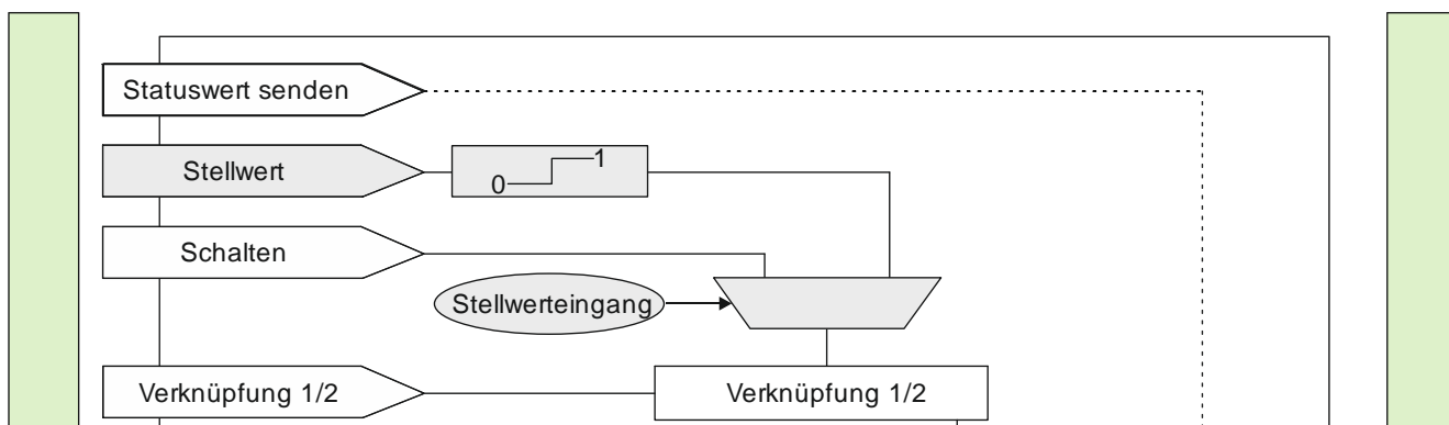
Abb. 7 Funktion Stellwerteingang
