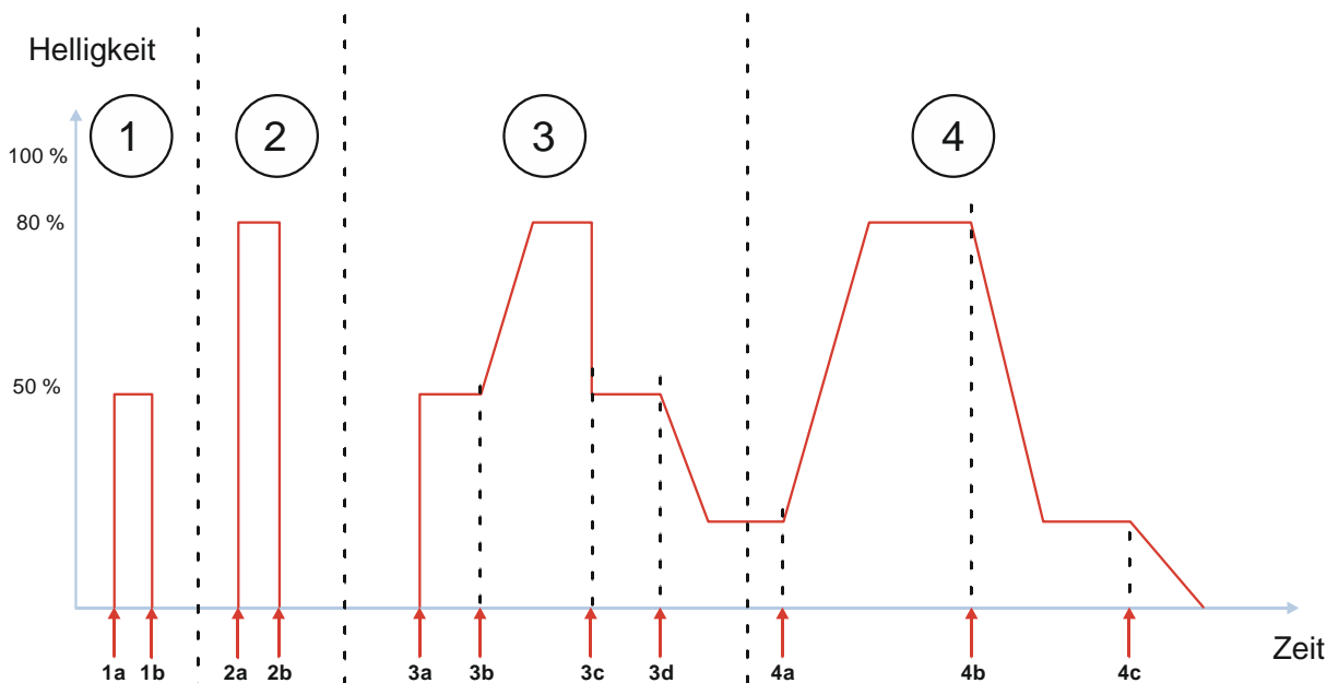
Abb. 51 Verhalten der Übersteuerungen des Kanals beim „Ein/-Ausschalten“ oder „Dimmen auf einen bestimmten Wert“ (Beispiel mit Übersteuerung „benutzerdefiniert“)
