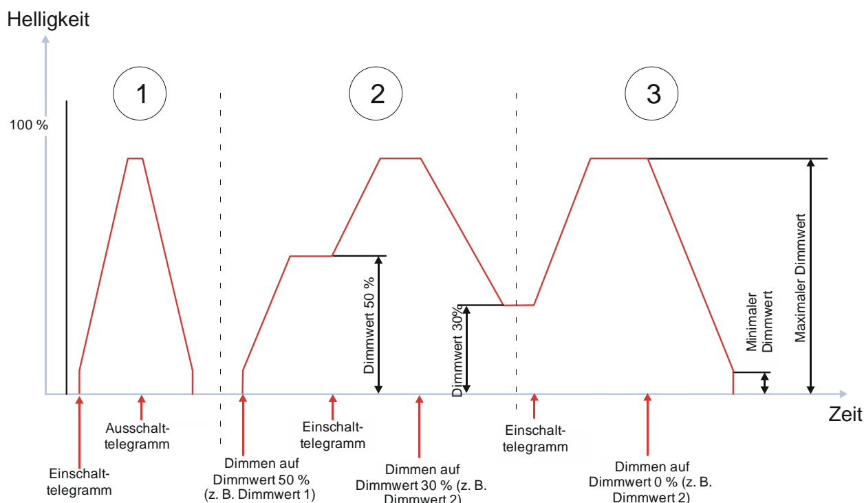
Abb. 34 Verhalten beim Einschalten und Dimmen auf einen Dimmwert unter Einfluss von minimalem und maximalem Dimmwert
