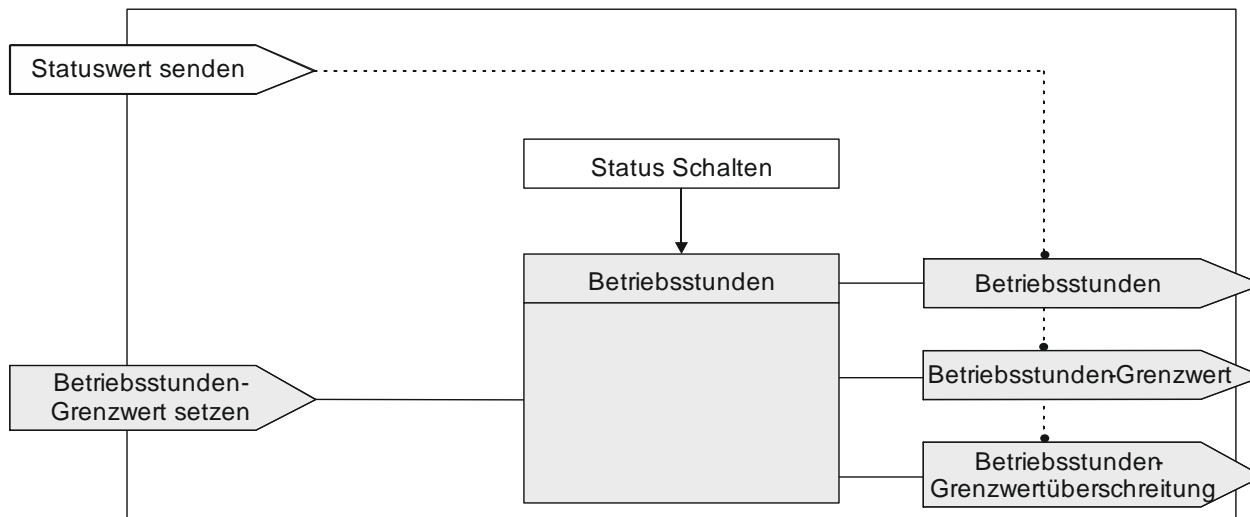
Abb. 22 Betriebsstundenzählung (Details)
