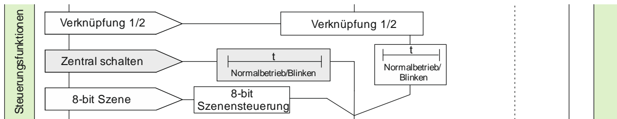
Abb. 8 Zentralschalten
