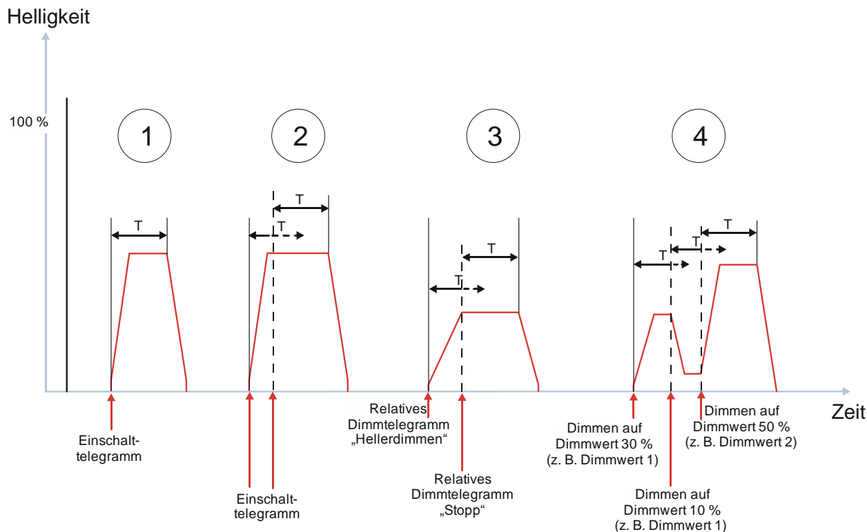
Abb. 38 Verhalten bei Zeitschalterbetrieb (1-fach) mit Einstellung „Nachtriggern = 1“
