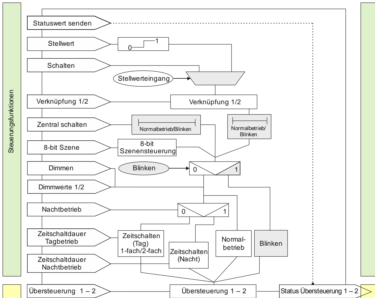
Abb. 5 Blinken
