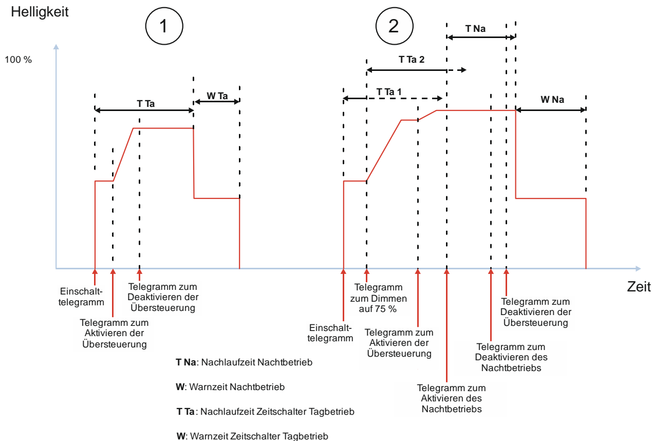
Abb. 53 Verhalten des Schalt-/Dimmkaktors im Zeitschalterbetrieb mit Nachtbetrieb, parametrierter Übersteuerung (Zwangsführung) und Vorgabe zum Neustart des Zeitschalters bei Deaktivierung der Übersteuerung
