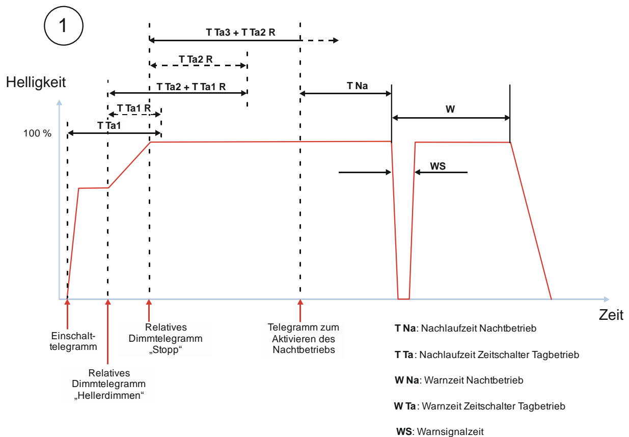
Abb. 47 Verhalten bei Aktivierung und Deaktivierung des Nachtbetriebs im Zeitschalterbetrieb (1-fach)
