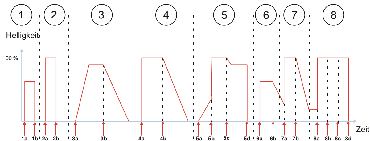
Abb. 50 Verhalten der Übersteuerungen des Kanals beim „Ein-/Ausschalten“ oder „Dimmen auf einen bestimmten Wert“ (Beispiel mit Übersteuerung „Hand EIN“)
