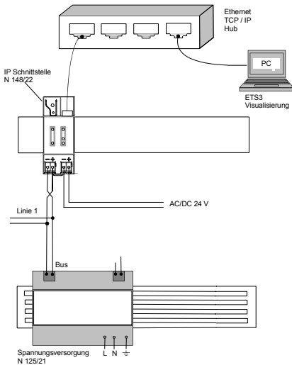
Anschlussbild 1 mit externer Hilfsspannungsversorgung Example of Operation 1 with external auxiliary power supply
