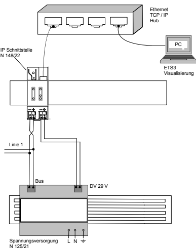
Anschlussbild 2 mit Hilfsspannungsversorgung aus unverdrosselter Busspannungsversorgung Example of Operation 2 with auxiliary power supply from unchoked bus power supply
