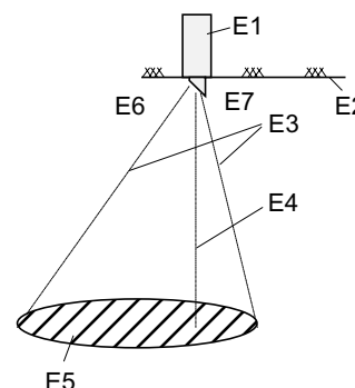
Bild 5: Montagehöhe GE 252
