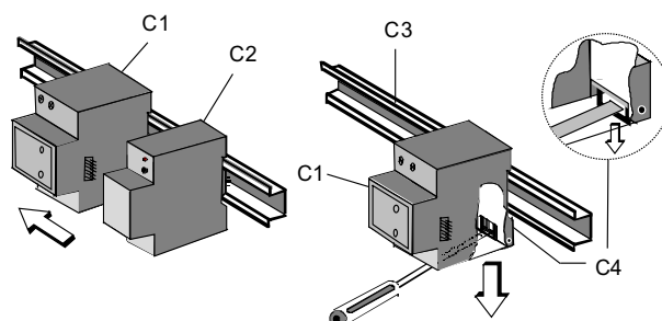
Bild 3: Demontage des Einbaugerätes
