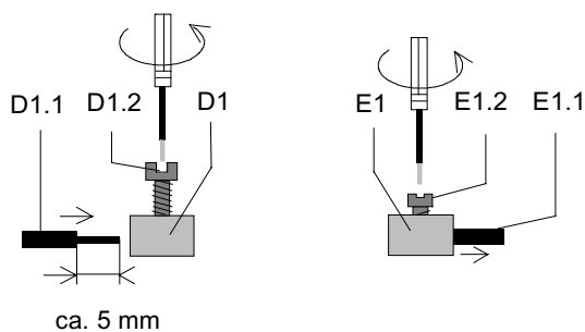
Bild 5: Anschlußleitung des Meßwertempfängers anschließen und abklemmen
