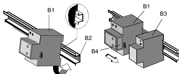
Bild 2: Montage des Einbaugerätes
