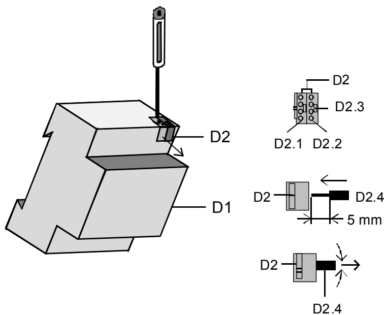
Bild 3: Busklemme aufstecken / entfernen
