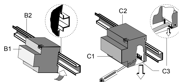
Bild 2: Montage / Demontage des Reiheneinbaugerätes
