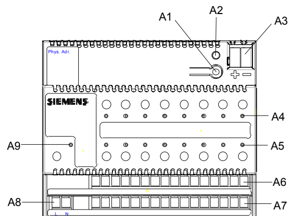
Bild 1: Lage der Anzeige- und Bedienelemente
