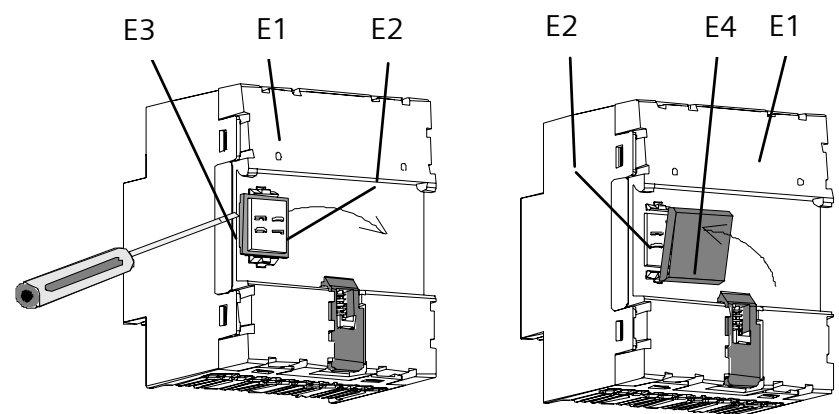
Bild 4: Abdecken des Kontaktsystems
