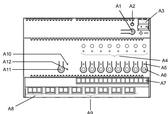
Bild 1: Lage der Anzeige- und Bedienelemente
