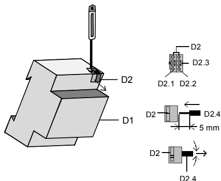
Bild 3: Busklemme aufstecken / entfernen
