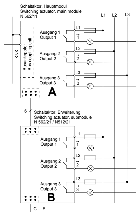
Bild 1. Anschlussbeispiel
