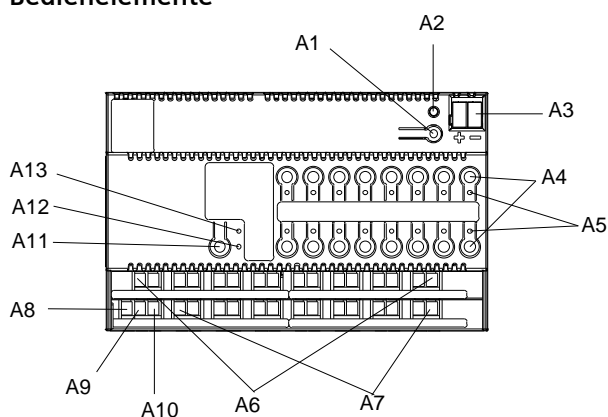
Bild 1: Lage der Anzeige- und Bedienelemente
