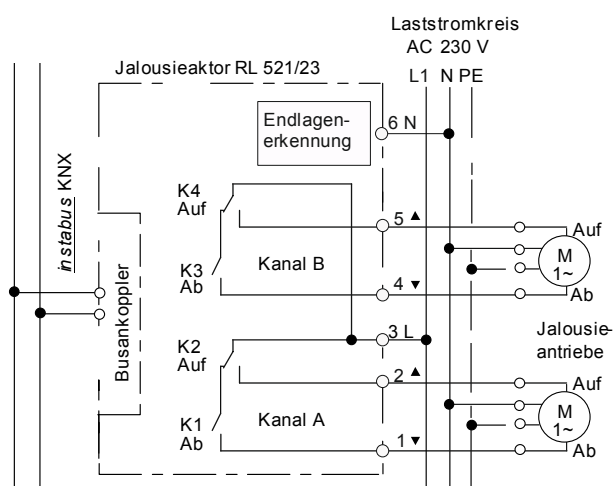
Bild 1: Anschlussbeispiel
