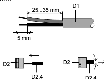
Bild 6: Busleitung anschließen / abklemmen
