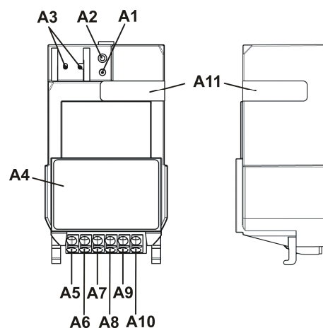
Bild 2: Lage- und Funktion der Anzeige- und Bedienelemente
