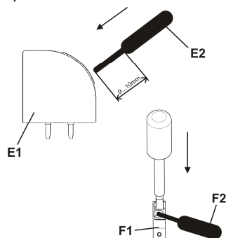
Bild 7: Netz- / Laststromkreis anschließen und abklemmen
