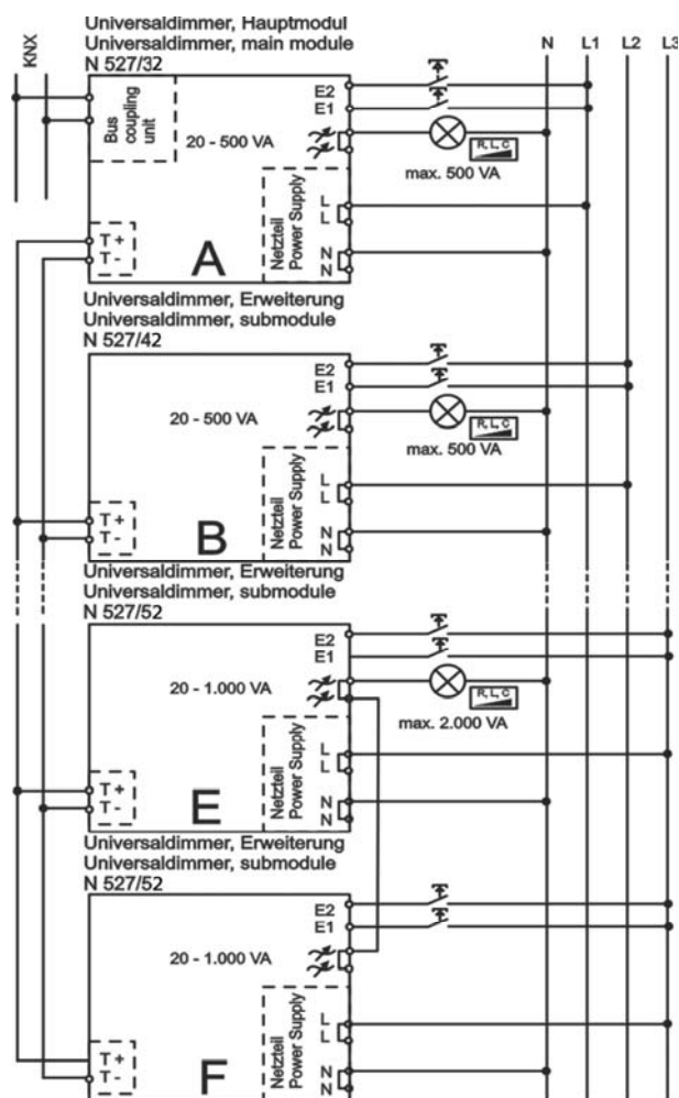
Bild 1. Anschlussbeispiel
