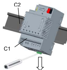
Bild 5. Demontage von einer Hutschiene
