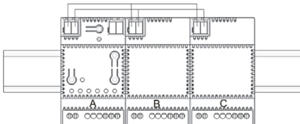
Bild 7. Verbinden von Universaldimmer-Erweiterungen
