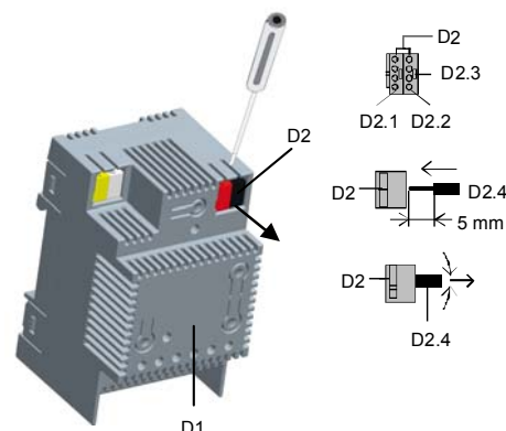
Bild 6. Klemmen aufstecken / entfernen
