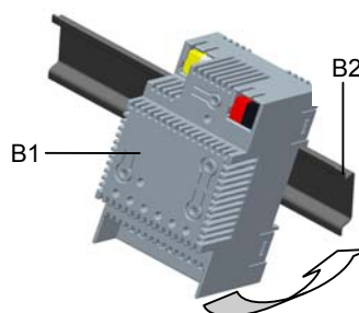
Bild 4. Montage auf einer Hutschiene
